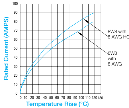
MCBX8W8 #8 Contacts
