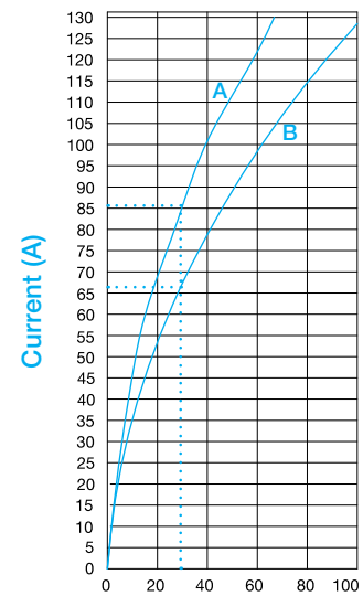
Size 4 Temperature rise (°C)
